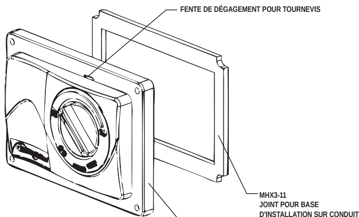
FIG. 2 INSTALLATION SUR CONDUIT
